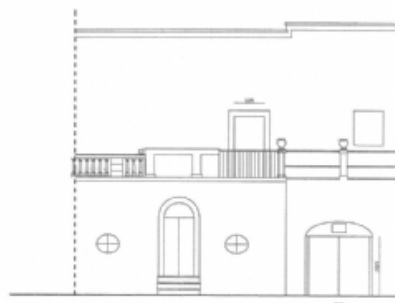
PROSPETTO LATERALE
