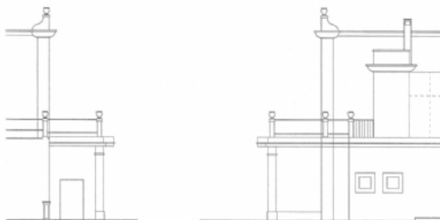
PROSPETTO LATI
